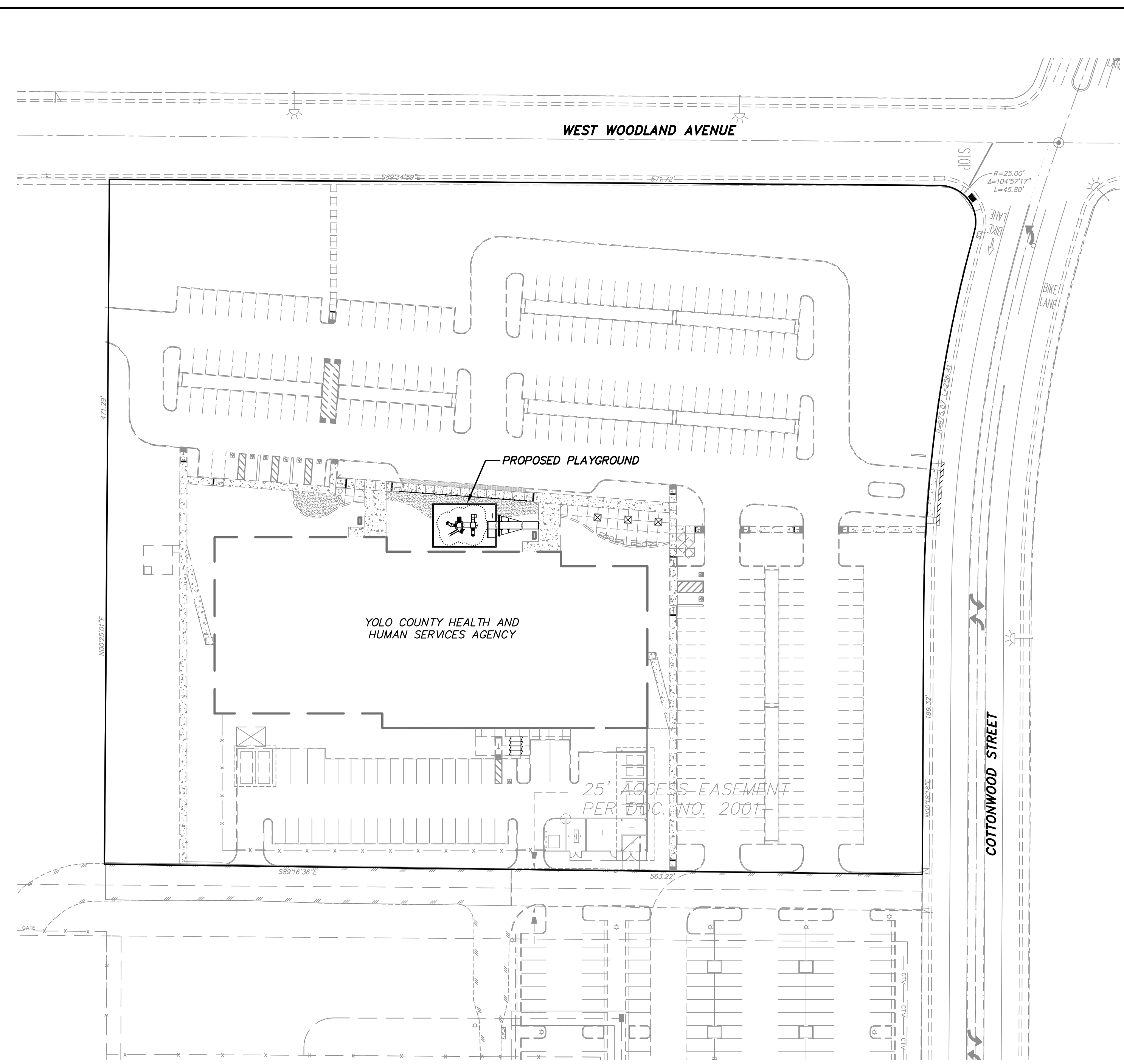
SITE PLAN NTS
